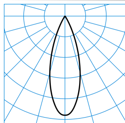
E-Line PRO 78 Lentyp L-FL 40-840 M35 ETBLE 05 05 TX716741
