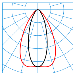
E-Line PRO 78IP50 MironaF T 130-840 ETDD L150 01 01 (LEO2) TX719970
