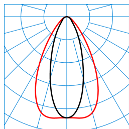
E-Line PRO 78IP50 MironaF T 130-840 ETDD L150 01 Blank (LEO1) TX719936
