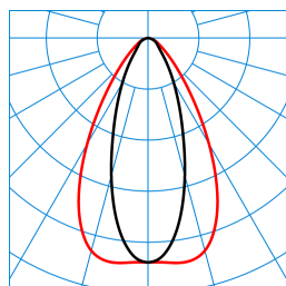
E-Line PRO 78IP50 MironaF T 130-840 ETDD L150 01 01 IP50 (LEO1) TX820885
