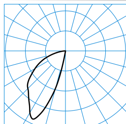
Linell 3PID5 WW-D-L 10-930 ETDD 01 TX829616
