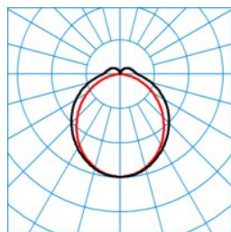
7850 DL35-100 ML 830 L150 12 50
