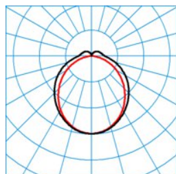
7850 DL35-100 ML 830 L150 14 50
