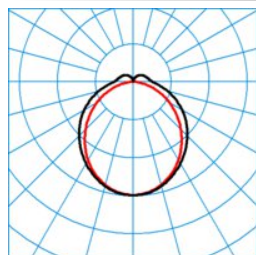
7850 DL35-100 ML 830 L150 10 50
