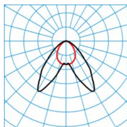
7850 LDAW40-110 ML 830 L150 10 50 ■ C0 - C180
