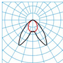
7850 LDAW40-110 ML 830 L150 14 50 ■ C0 - C180
