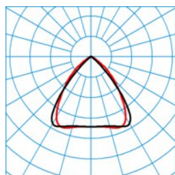
7850 LN40-110 ML 830 L150 10 50
