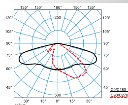
LnPlus 40-AB7L-SLR1/13500-727 12G1 ET (CLO initial value)
