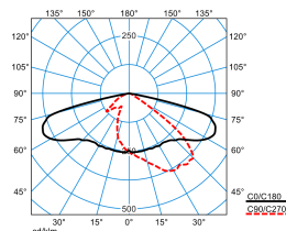
LnPlus 40-AB7L-SLR1/13500-727 12G1 ET (CLO end value)
