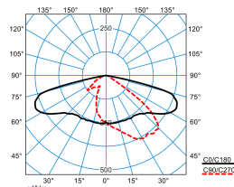
LnPlus 60-AB7L-SLR1/24000-727 18G1 ET (CLO end value)
