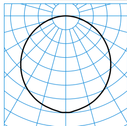
Varisto600 6000-840 S09 ET 01 TX843046
