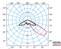
LnPlus 40-AM19L-SLR2/13500-727 12G1 ET (CLO end value)
