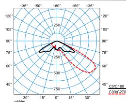
LnPlus 40-AM19L-SLR2/13500-727 12G1 ET (CLO initial value)
