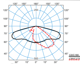
LnPlus 40-AB7L-SLR3/13500-740 12G1 ET (CLO initial value)
