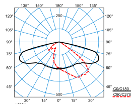
LnPlus 40-AB7L-SLR3/13500-740 12G1 ET (CLO end value)
