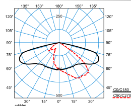
LnPlus 40-AB7L-SLR3/15000-727 12G1 ET (CLO initial value)
