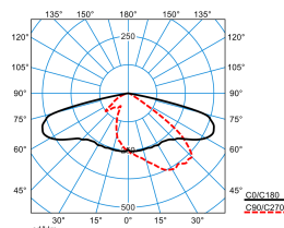
LnPlus 40-AB7L-SLR3/15000-730 12G1 ET (CLO end value)
