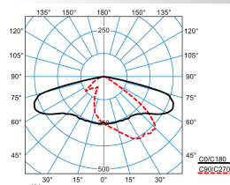
LnPlus 40-AB7L-SLR3/15000-730 12G1 ET (CLO initial value)
