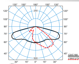
LnPlus 60-AB7L-SLR3/29000-740 24G1 ET (CLO initial value)
