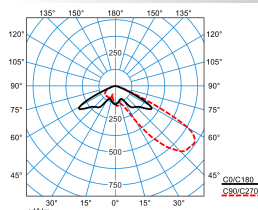
LnPlus 70-AM19L-SLR3/38000-740 36G1 ET (CLO initial value)
