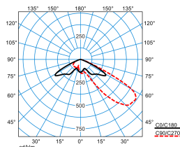
LnPlus 70-AM19L-SLR3/38000-740 36G1 ET (CLO end value)
