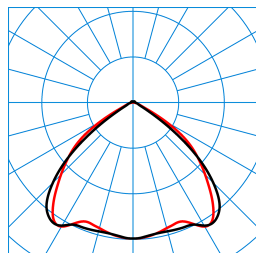
E-Line B LED4000-865 IP54 TX053205
