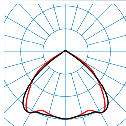
7650B LED8000-840 ET 05 TX784323
