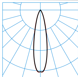
7650 G2 T LED20000-865 ETDD TX719633
