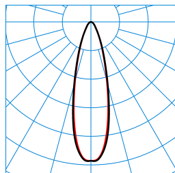
E-Line T LED4000-865 IP54 TX053411
