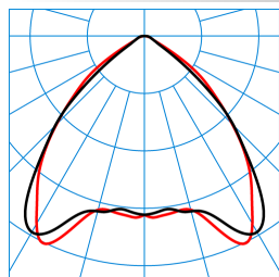
7650 G2 TB LED13000-840 ET TX784515
