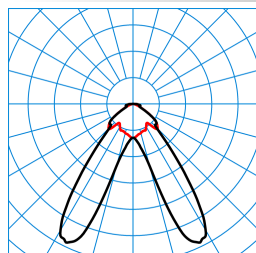
7650DA LED8000-865 ET TX784565
