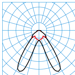
E-Line DA LED8000-865 IP54 TX053250
