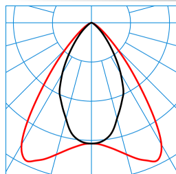
7650M-MT LED4000-865 ET TX719654
