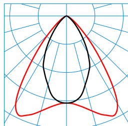
E-Line M-MT LED4000-865 IP54 TX053315
