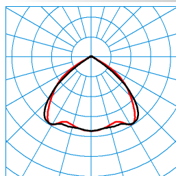
E-Line G2 B LED10000-840 TX054366
