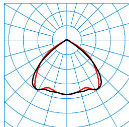
E-Line G2 B LED10000-840 IP54 TX370958
