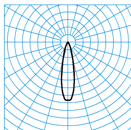
E-Line G2 M-T LED10000-840 IP54 TX370263
