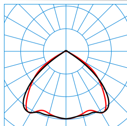
7650 G3 M-B LED10000-840 ET TX784289
