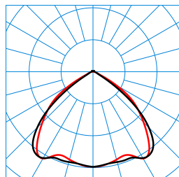
E-Line G2 M-B LED10000-840 IP54 TX054554
