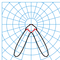
E-Line G2 M-DA LED10000-830 IP54 TX054556
