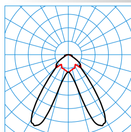
7650 G3 M-DA LED10000-830 ET TX784263
