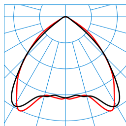
E-Line G2 TB LED10000-865 IP54 TX054576
