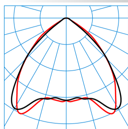
7650 G3 TB LED10000-865 ET TX784283
