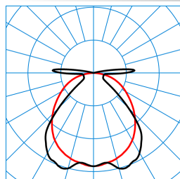
OleveonF 15 B 6000-840 ET PC TWS TX782685
