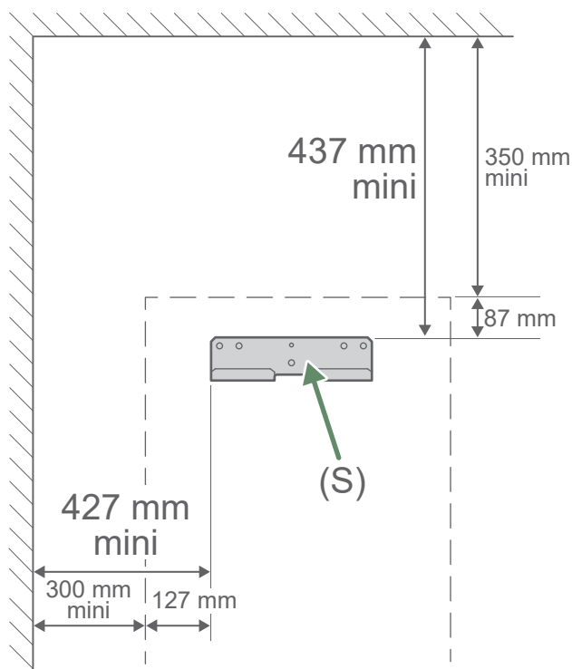
fig. 21 - Fixation murale
