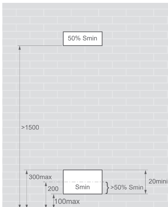
fig. 24 - Position des ouvertures pour la ventilation
