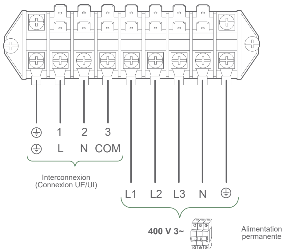
fig. 41 - Borniers de raccordement électrique coté unité extérieure
