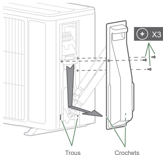
fig. 12 - Ouverture de l'unité extérieure modèles 5, 6 et 8
