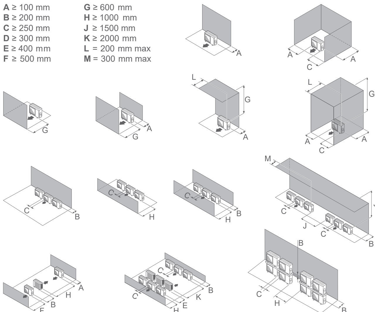
fig. 15 - Dégagements minimum d'installation autour de l'unité extérieure
