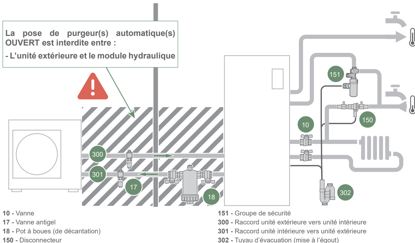
fig. 9 - Raccordements
