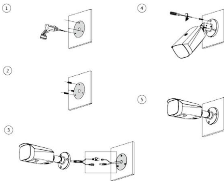
Figure 3-3. Passage du câble à travers la surface de montage•
