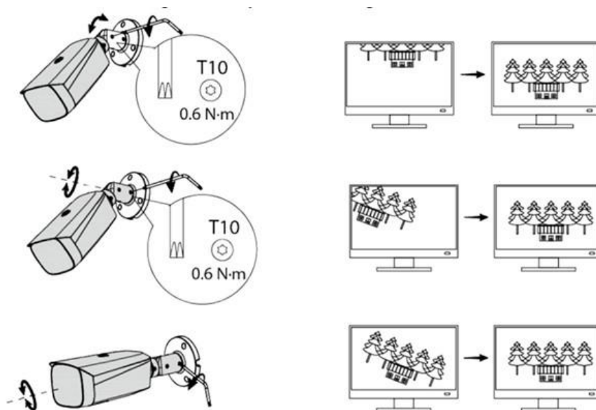
Figure 3-6. Réglage de l'angle de l'objectif
