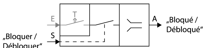
Image 22: Représentation schématique de la « fonction de blocage »
