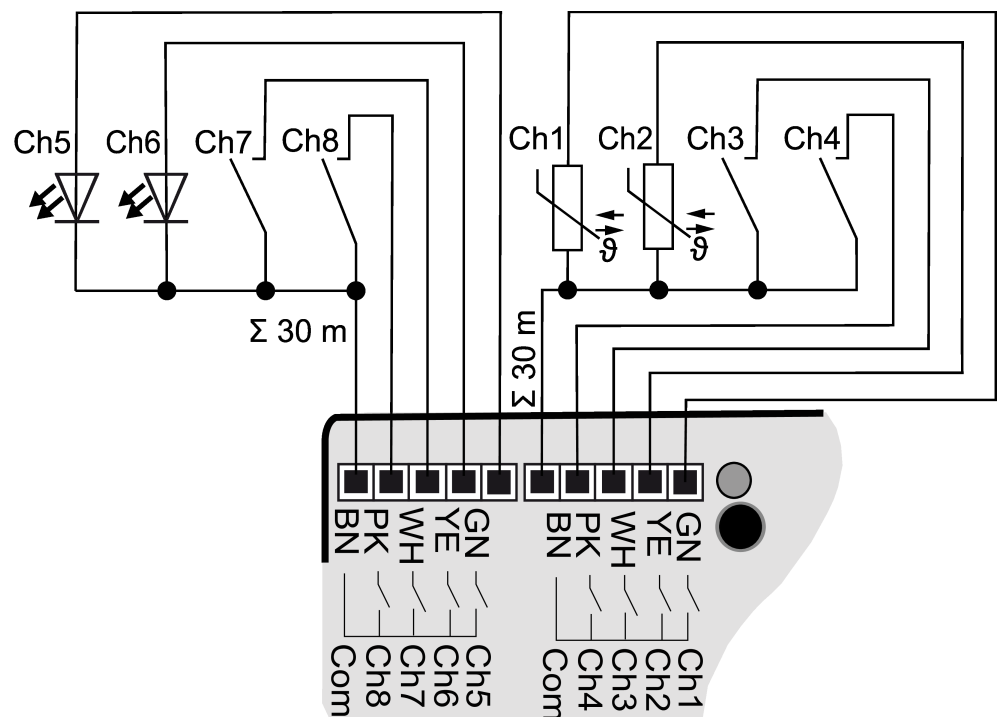
Image 6: Exemple de raccordement avec des sorties en parallèle
