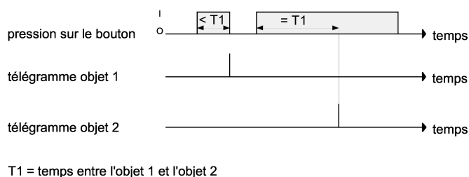
Image 11: Exemple de concept de commande « Objet 1 ou objet 2 »
