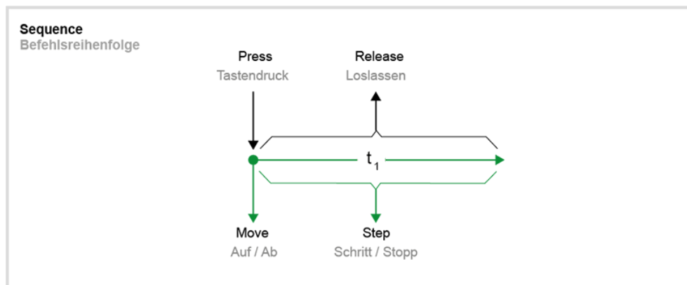
Image 8: Concept de commande « Haut/bas - Pas à pas »
