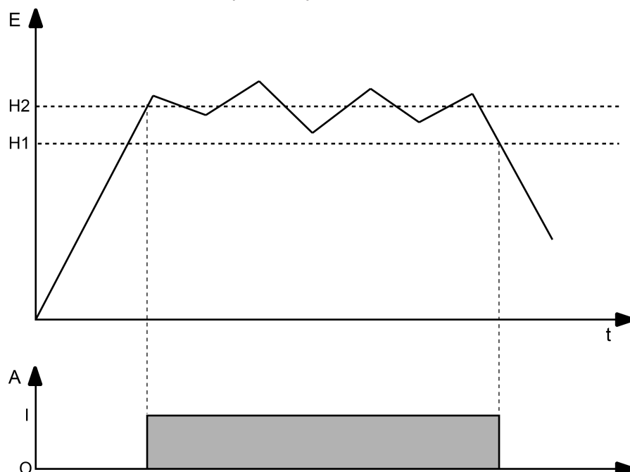
Image 28: Exemple d'une évaluation d'hystérésis grâce à la valeur seuil supérieure et à la valeur seuil inférieure
