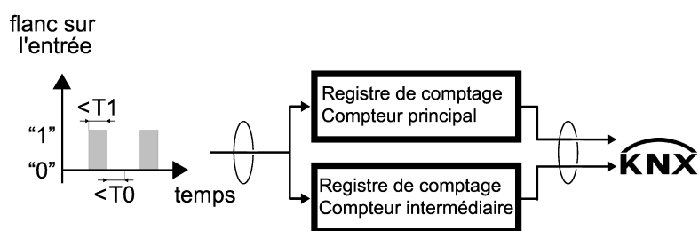
Image 13: Schéma fonctionnel du compteur d'impulsions
