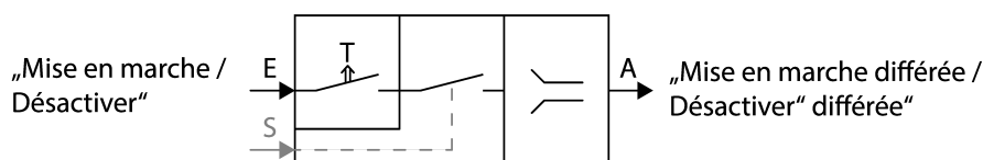
Image 20: Représentation schématique « Enclenchement et déclenchement temporisés »
