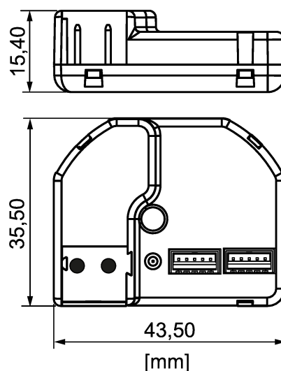
Image 2: Schéma coté
