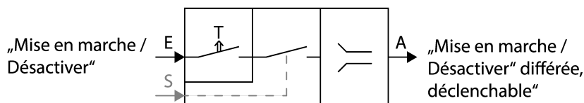
Image 21: Représentation schématique « fonction cage d'escalier »
