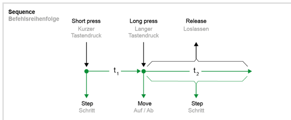
Image 7: Concept de commande « Pas à pas Haut / Bas - Pas à pas »
