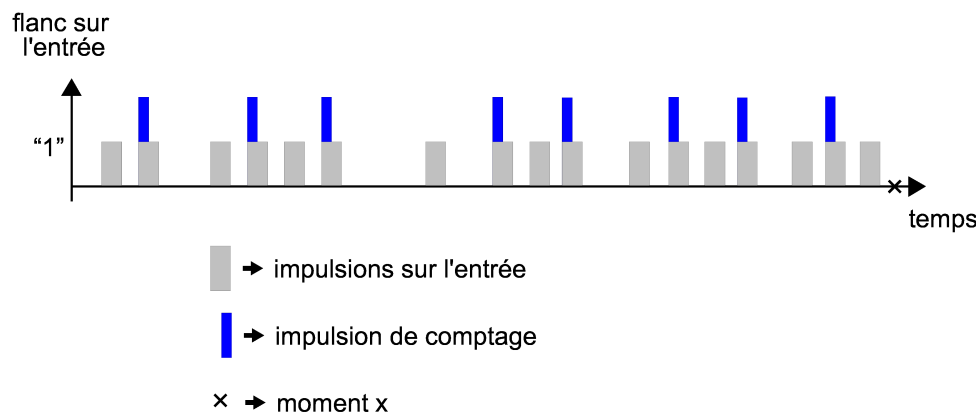
Image 15: Exemple de réglage des modifications de l'état du compteur par impulsion de comptage
