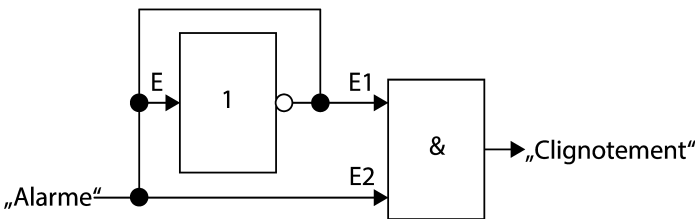
Image 17: Représentation schématique « clignotement »
