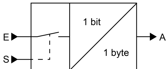
Image 24: Convertisseur (1 bit -> 1 octet)
