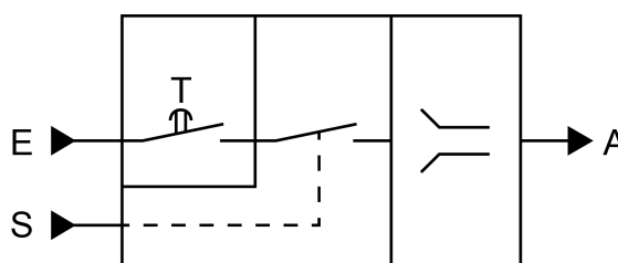
Image 25: Élément de blocage (filtre/temps)
