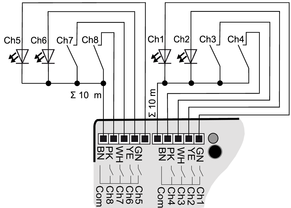
Image 5: Exemple de raccordement de l'interface de bouton-poussoir octuple
