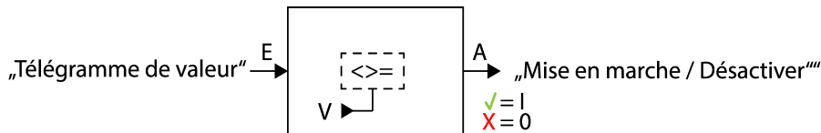
Image 23: Représentation schématique « Affichage de l'état de la valeur de comparaison
