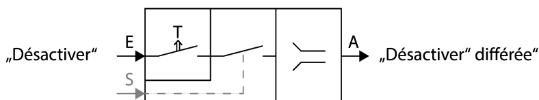
Image 19: Représentation schématique « Arrêt différé »
