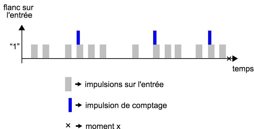
Image 14: Exemple de réglage des impulsions sur l'entrée par impulsion de comptage
