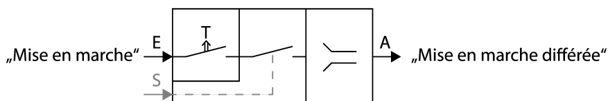
Image 18: Représentation schématique « Enclenchement retardé »
