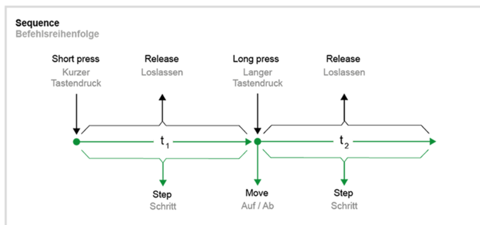
Image 10: Concept de commande « haut/bas - pas ou pas »
