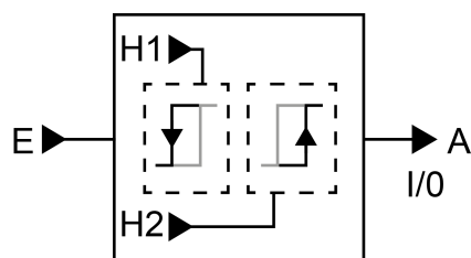
Image 27: Commutateur à valeur limite
