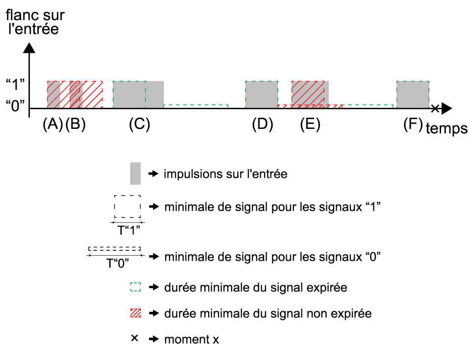
Image 16: Exemple de réglage de la durée minimale de signal
