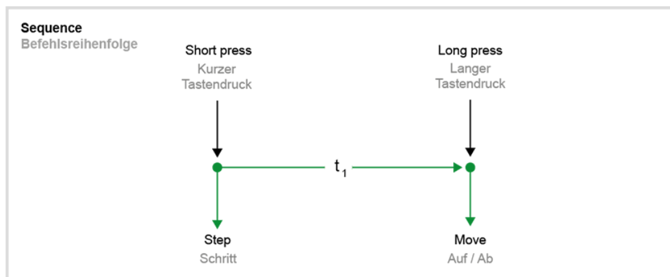
Image 9: Concept de commande « pas à pas - haut/bas »
