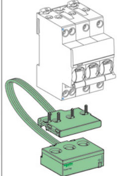
A9MEM1572 - 3P+N Un 230/400 V~
