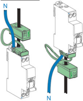
1P+N - Un 230 V~
