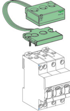
A9MEM1571 - 3P+N Un 230/400 V~
