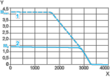
Courbes couple/vitesse Servomoteur avec servovariateur LXM32•D18M2
