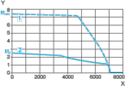
Courbes couple/vitesse Servomoteur avec servovariateur LXM32•D12N4
