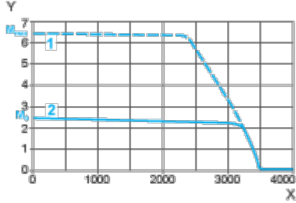
Courbes couple/vitesse Servomoteur avec servovariateur LXM32•D30M2
