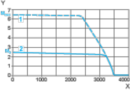
Courbes couple/vitesse Servomoteur avec servovariateur LXM32•D30M2
