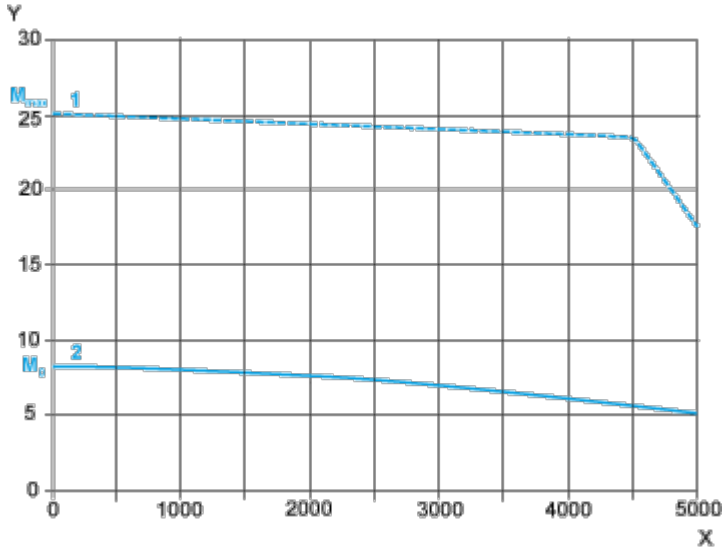
Courbes couple/vitesse Servomoteur avec servovariateur LXM32•D30N4
