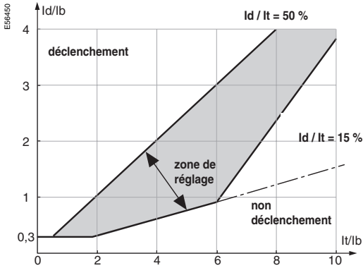
Caractéristique de fonctionnement en pourcentage
