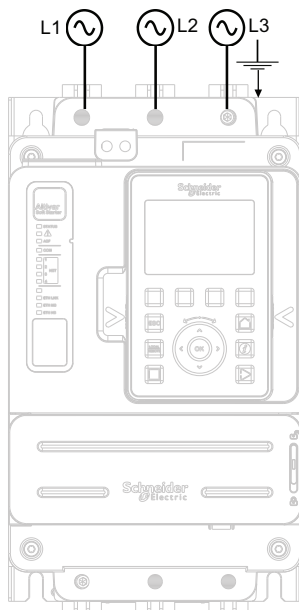
Côté réseau
