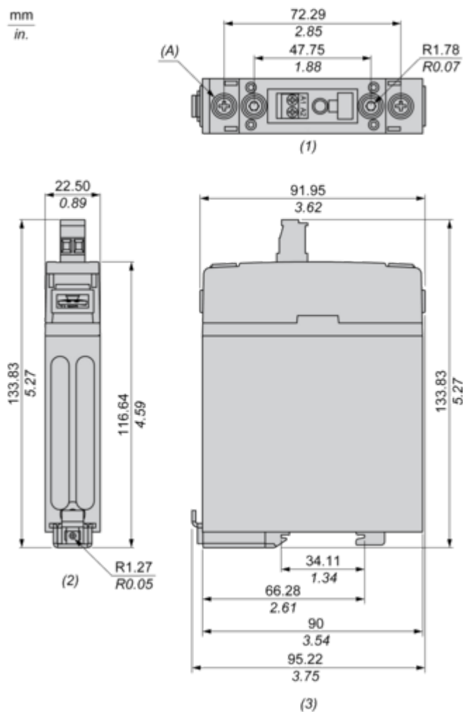
(1) Vue de face (2) Vue du dessus (3) Vue latérale (A) Vis 8-32 à profil rehaussé par plot 1/4 48 UNS (2 emplacements)
