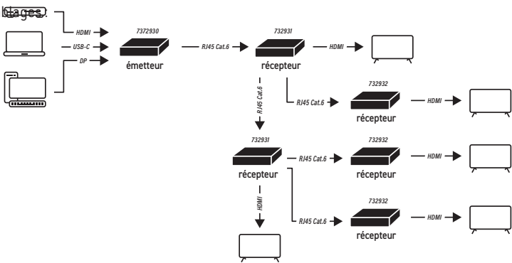
Schéma de câblages
