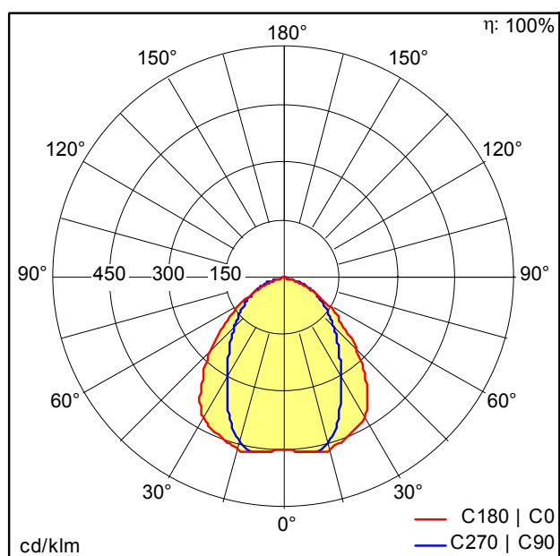
D46288AA_TRINOS_10000-865_L2000_VWB_LDE_WH.Idt
