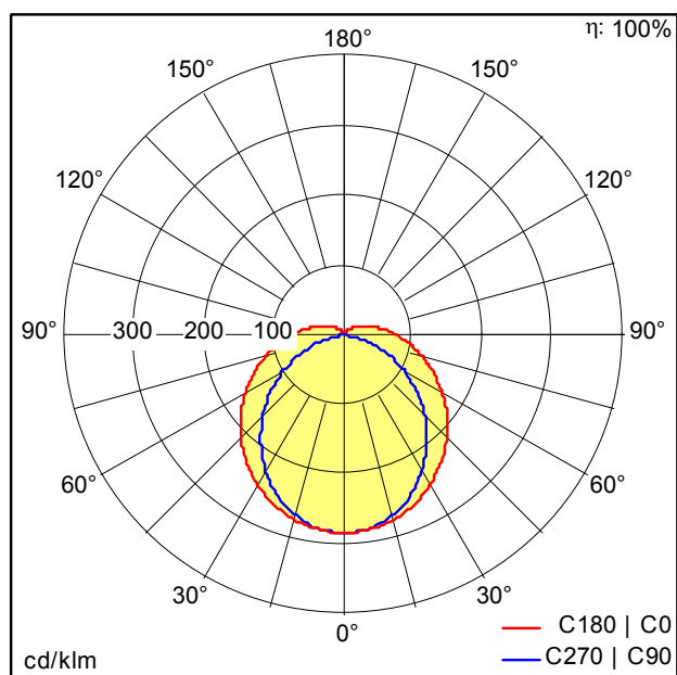
TLX_HO_6200-840_O_SMID_L.Idt
