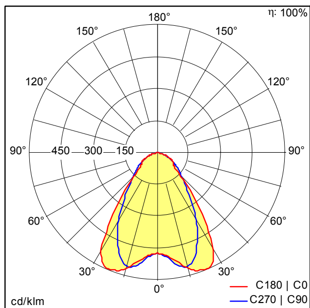
D44421AA_TEC_LED8000-840_L1000_WB_LDE_SR_IP.idt
