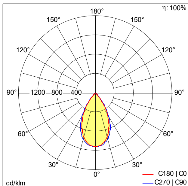
Sceno_(2x7)_4000-835-wfl_re.Idt, Sceno_(2x7)_4000-835-wfl_li.Idt
