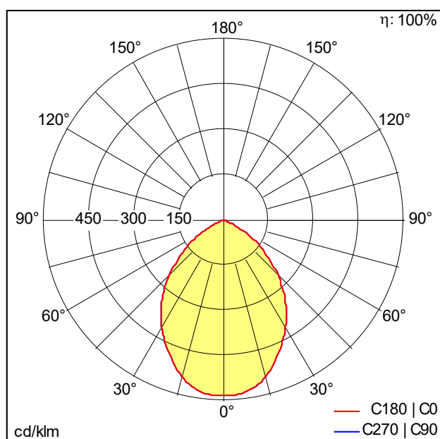
PANOS_R_R_200_2k-940_SWI_L_FAL_WH.Idt
