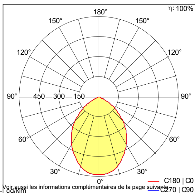
PANOS_R_R_200_4k-840_LDO_L_FAL_WH.Idt
